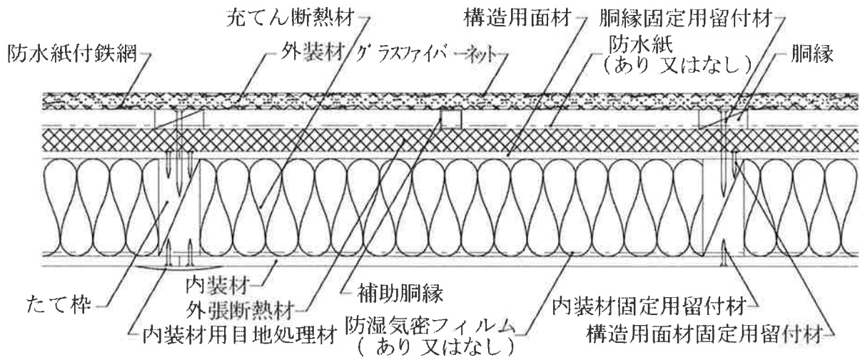
水平断面図
