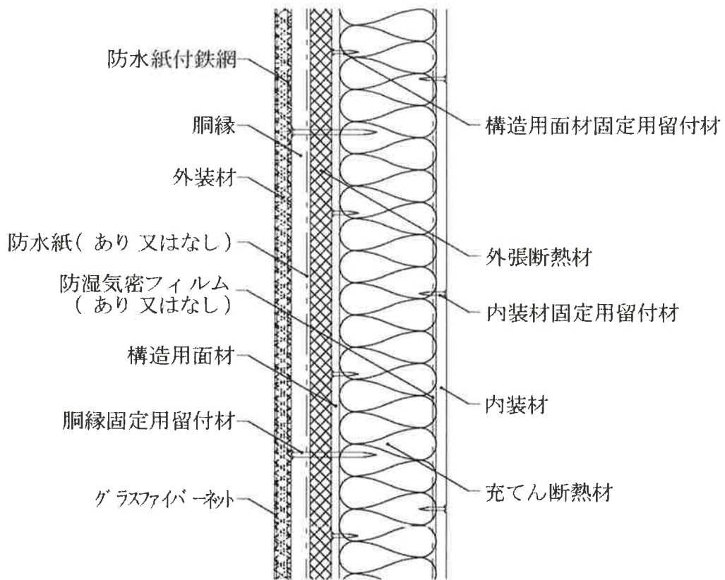
鉛直断面図
