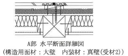
A部 水平断面詳細図 (構造用面材：大壁 内装材：真壁(受材1))
