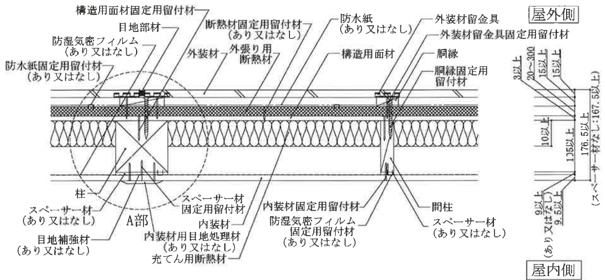
水平断面詳細図 (構造用面材・内装材：大壁)
