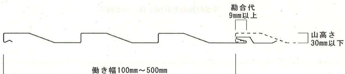
外装材断面形状図：Ⅳ．勘合式
