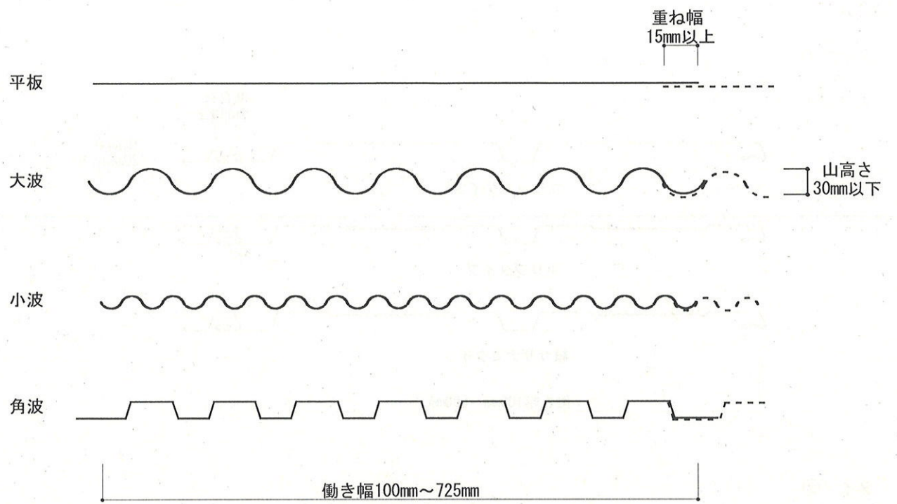
外装材断面形状図：Ⅱ．重ね式
