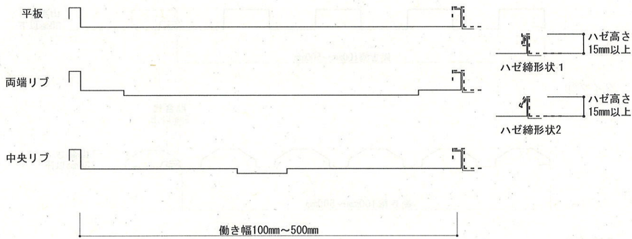
外装材断面形状図：Ⅲ．ハゼ締式
